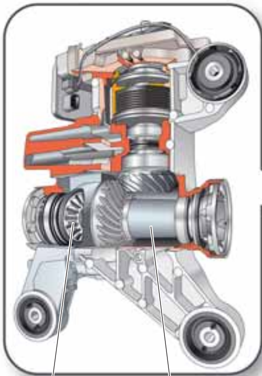
Haldex-Kupplung 02D/0AV
